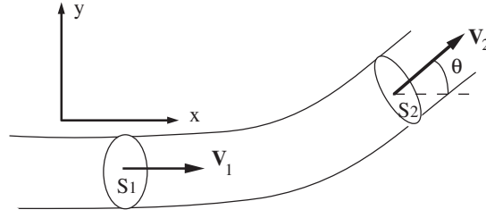
Figure 8.8: Ecoulement dans une conduite coudée.
