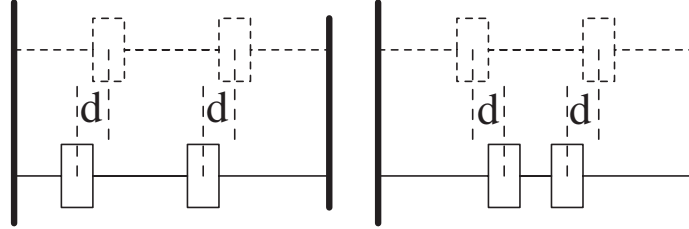
Figure 1.8: Modes propres du système de la Fig. 1.7. Les dessins en pointillés représentent l'état d'équilibre, ceux en traits pleins le mouvement à un instant donné. A gauche, les deux oscillateurs sont en phase, à droite en opposition de phase.
