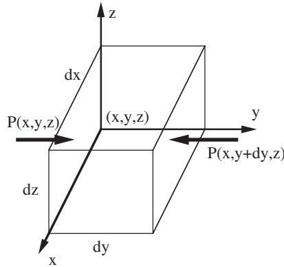
Figure 8.2: Volume élémentaire de fluide à l'équilibre.
