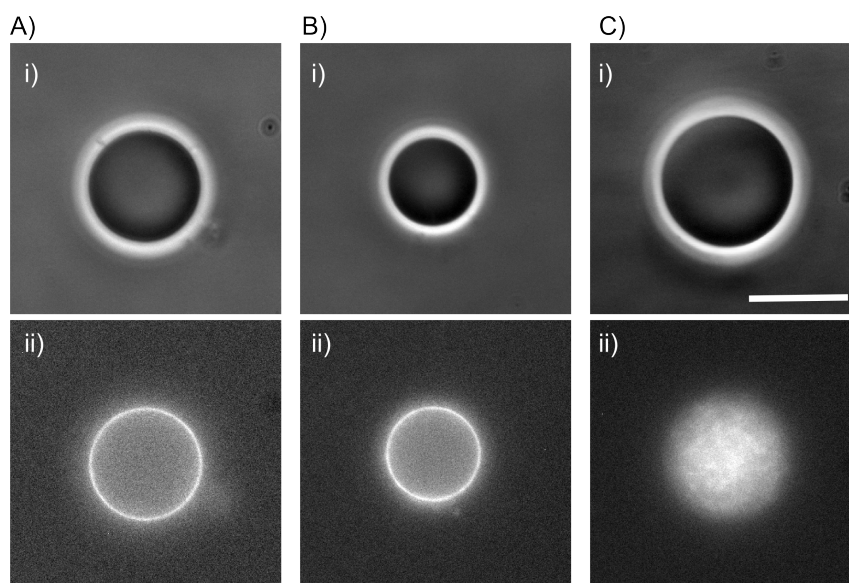
FIGURE 5.5 – Effet de la CP sur le réseau d’actine polymérisée à la surface d’un liposome. La concentration en CP est indiquée au dessus des images, en épifluorescences, des liposomes recouverts d’actine fluorescente. En dessous est tracé le profil d’intensité le long de la ligne jaune traversant les liposomes. Plus la concentration de CP est élevée et plus le réseau est fin. Echelle 10 \mu\text{m} .
